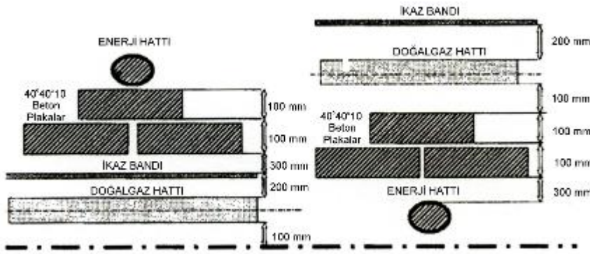
Şekil 5 — Doğal gaz hattı ile elektrik kabloları arasındaki mesafe
