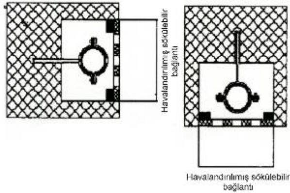
Şekil 7 — Duvar/Asma tavan içi kanal ve boru geçiş detayı
