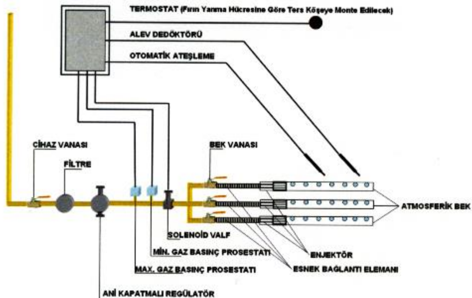
Şekil 18 — Fırınlarda brülör emniyet ekipmanları montaj şeması
