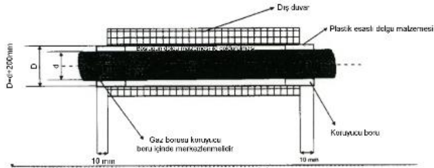
Şekil 6 — Duvar Geçişi
