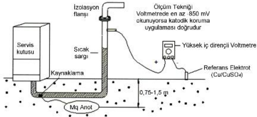
Şekil 8 — Katodik Koruma
