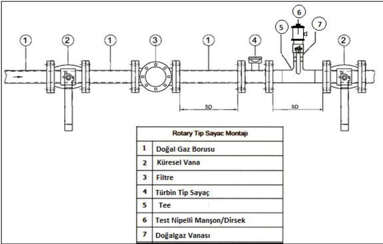
Şekil 11 — Türbinli sayaçlara ait bağlantı detayı
