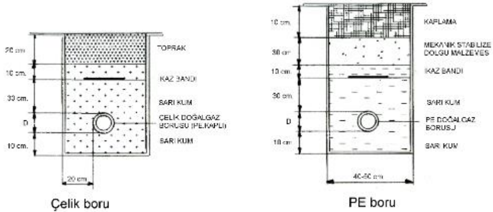
Şekil 3 — Toprak altı hat ayrıntıları
