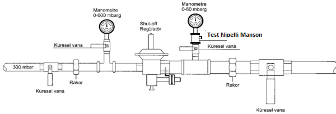
Şekil 12 — Konut tipi regülatör bağlantısı
