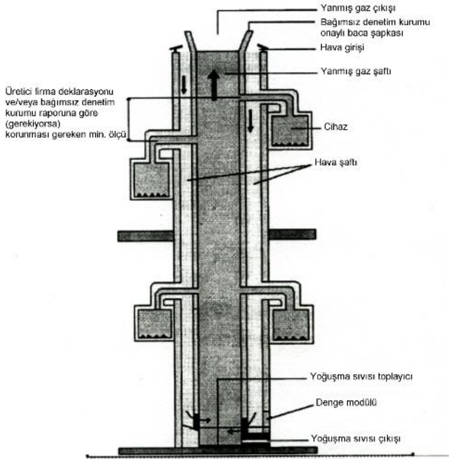
Şekil 25 - Hava-atık gaz baca sistemleri
