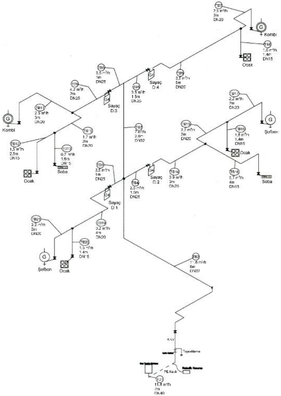
Şekil 1 — Örnek 1'e ait izometrik kolon şeması
