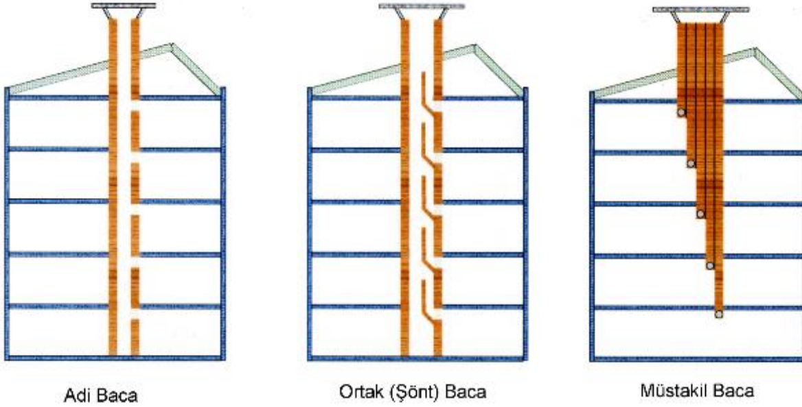
Şekil 23 — Bacalar
