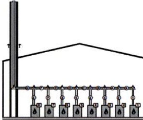
Şekil 16 — Kaskad baca sistemi
