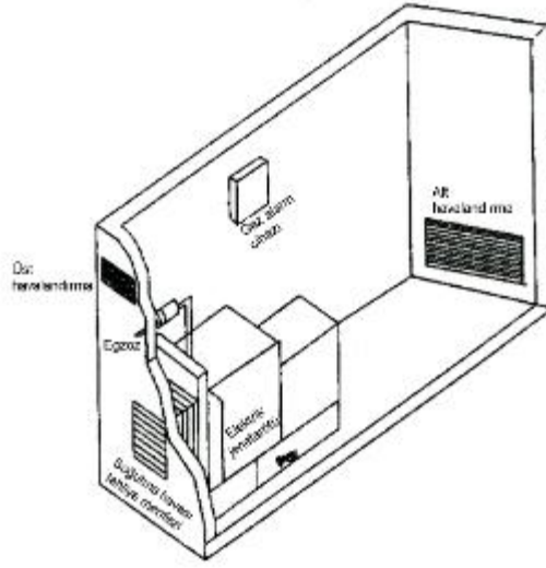
Şekil 17 — Elektrik jeneratör dairesi
