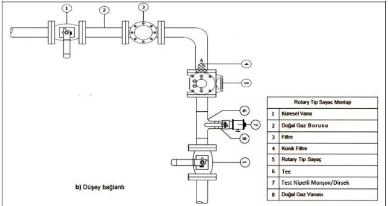
Şekil 10 — Rotary sayaçlara ait bağlantı detayı
